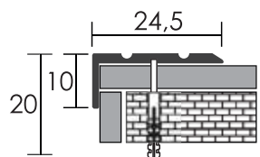
Pravouhý schodový profil – vrtaný, hliník
